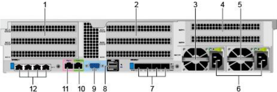
图 4-4 后面板组件
