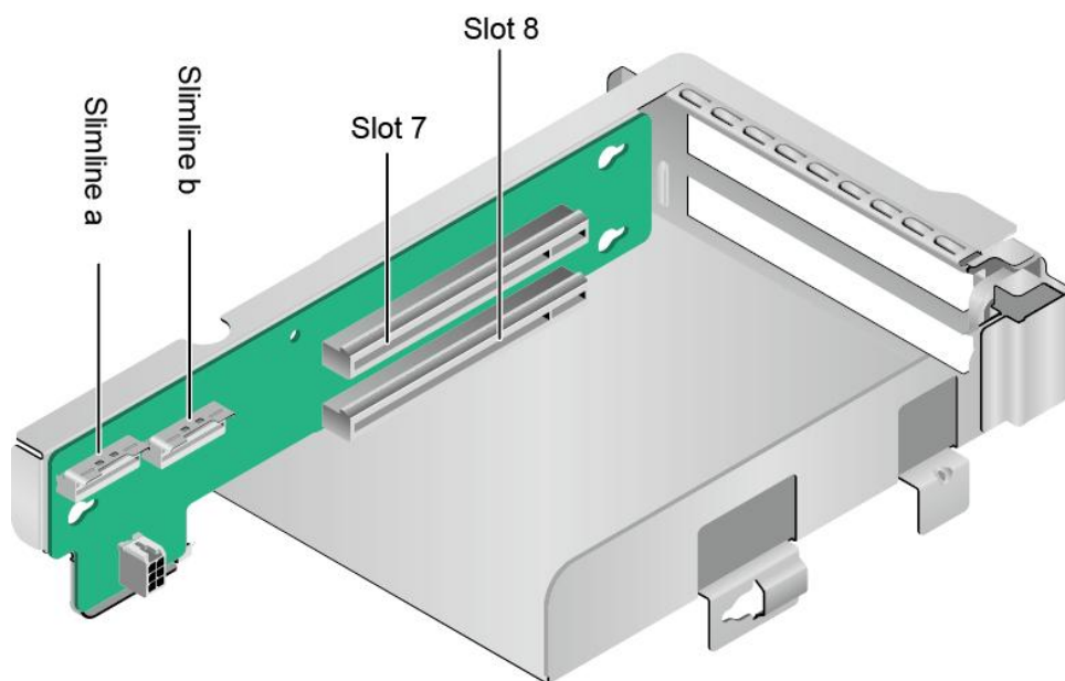
图 4-17 Riser 卡 6 (2x8)
