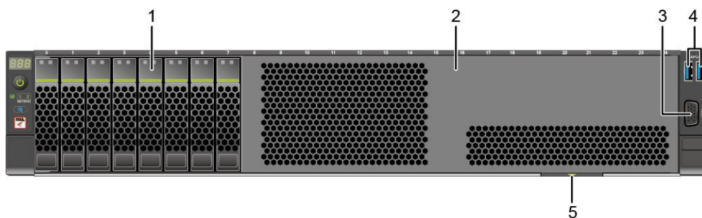
图 4-3 8x2.5 英寸硬盘配置前面板组件
