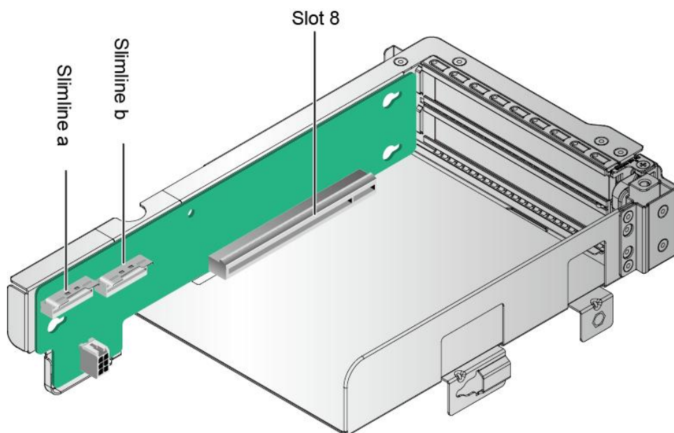
图 4-18 Riser 卡 7 (1x16)
