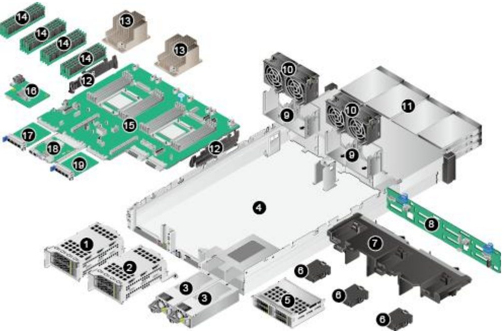
图 4-20 部件
