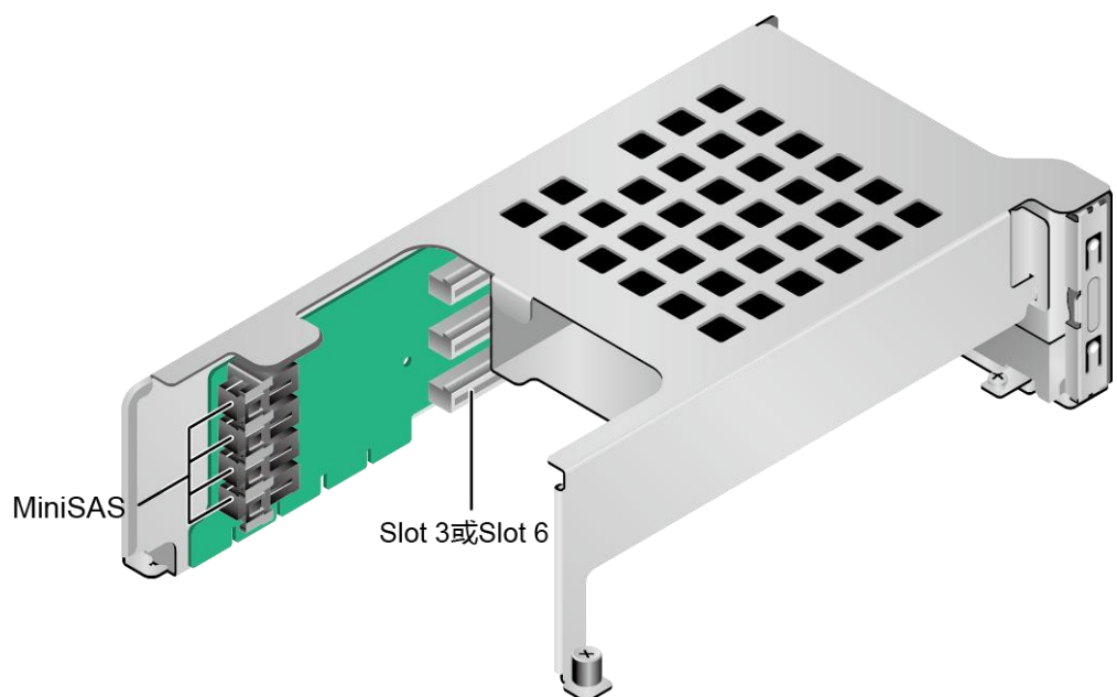
图 4-16 SAS Riser 卡 5
