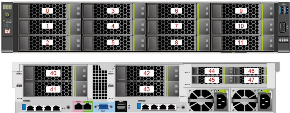
图 6-3 12x3.5 英寸 EXP 硬盘配置
