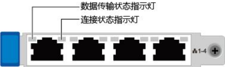
图 4-11 TM210（4*GE 电口）
