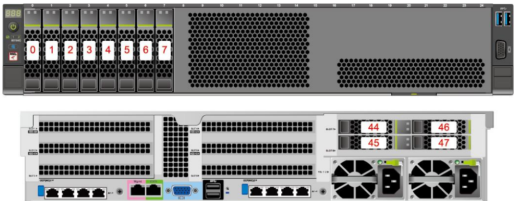
图 6-6 8x2.5 英寸硬盘配置的硬盘编号
