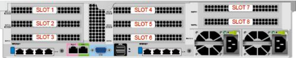
图 4-19 PCIe 插槽
